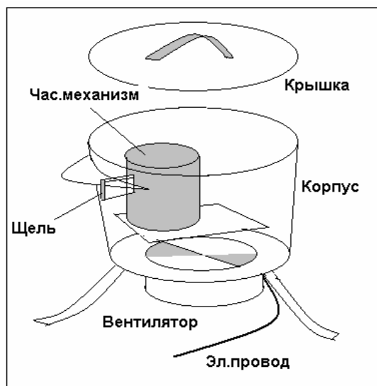
Рисунок 1 – Схема ловушки
